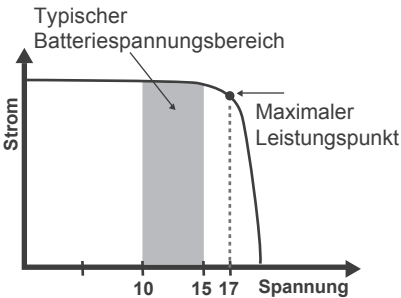
Strom und Spannung (12V-System)
