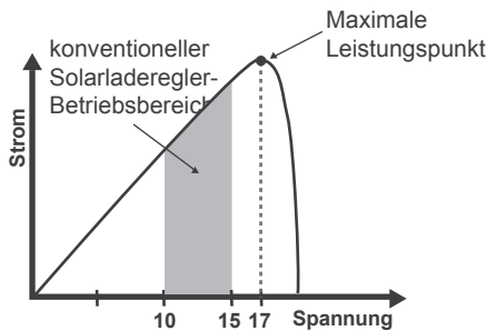
Ausgangsleistung (12V-System)
